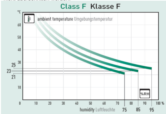
Grenzen der relativen Luftfeuchte des Kondensators in Abhängigkeit von der Umgebungstemperatur. Limits of relative humidity of the ambient climate in relation to the ambient temperature.
